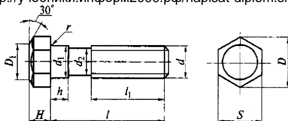
Рис. 18.2. Параметры, определяющие размеры болта
