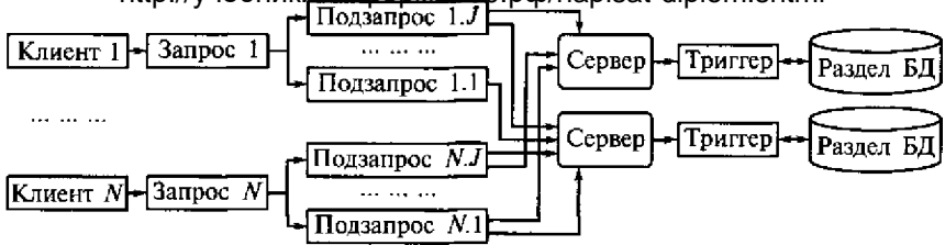
Рис. 10.13. Схема выполнения запроса при смешанном параллелизме
