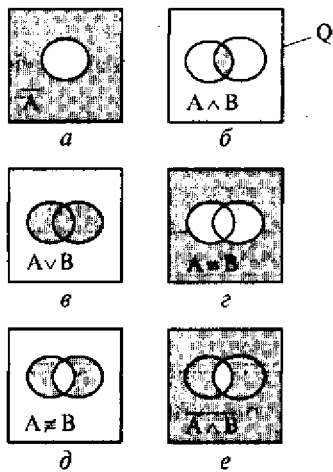
Рис. 1.4. Графическое изображение булевых функций: a — множество A ; b — пересечение множеств; c — объединение множеств; d — эквивалентности двух множеств; e — отрицание эквивалентности; e — отрицание конъюнкции
